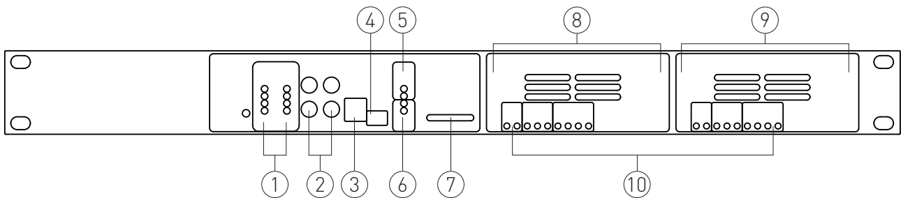
Abbildung 1 Anschlussbezeichnung Vorderansicht
