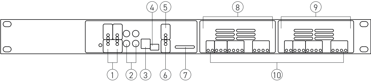
Abbildung 1 Anschlussbezeichnung Vorderansicht
