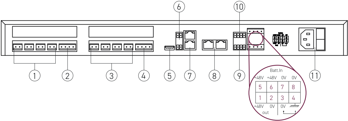
Abbildung 2 Anschlussbezeichnung Rückansicht
