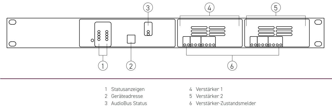
Abbildung 1 Anschlussbezeichnung Vorderansicht
