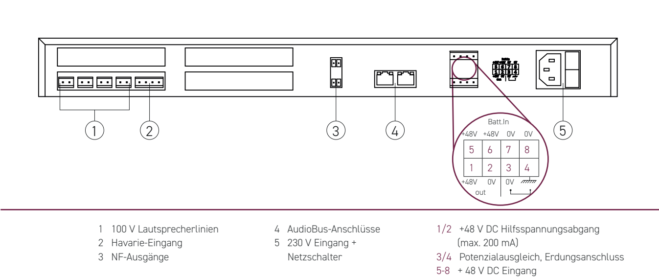
Abbildung 2 Anschlussbezeichnung Rückansicht
